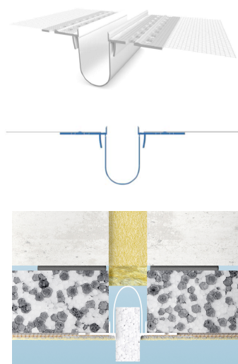
Capatect Dehnfugenprofil Plus 6660/00 Typ E
