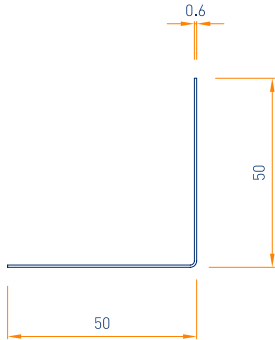
vista frontale scala 1:2
