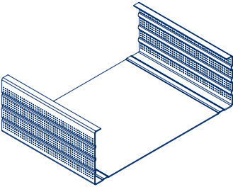
assonometria scala 1:5
