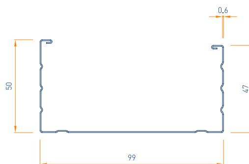
vista frontale scala 1:2
