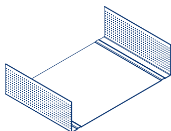
assonometria scala 1:5
