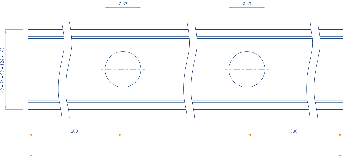
vista in pianta forature profilo scala 1:2
